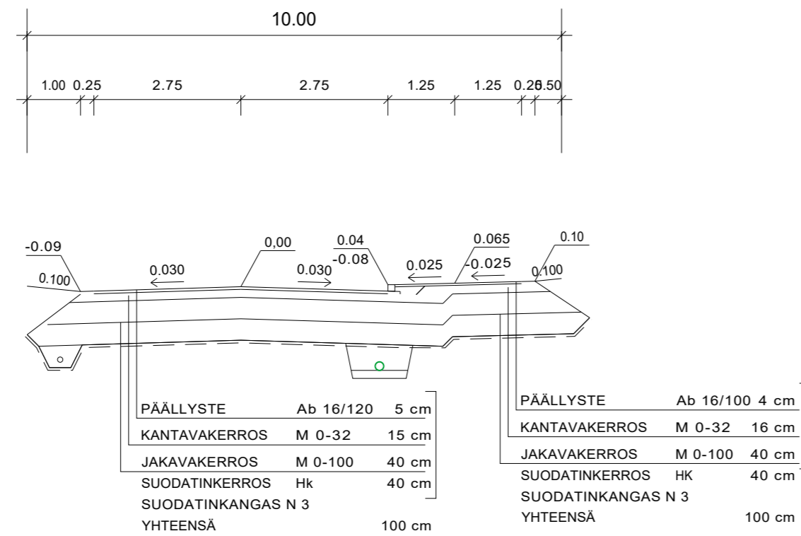
TYYPPIPOIKKILEIKKAUS PAALULTA 120 1:100
