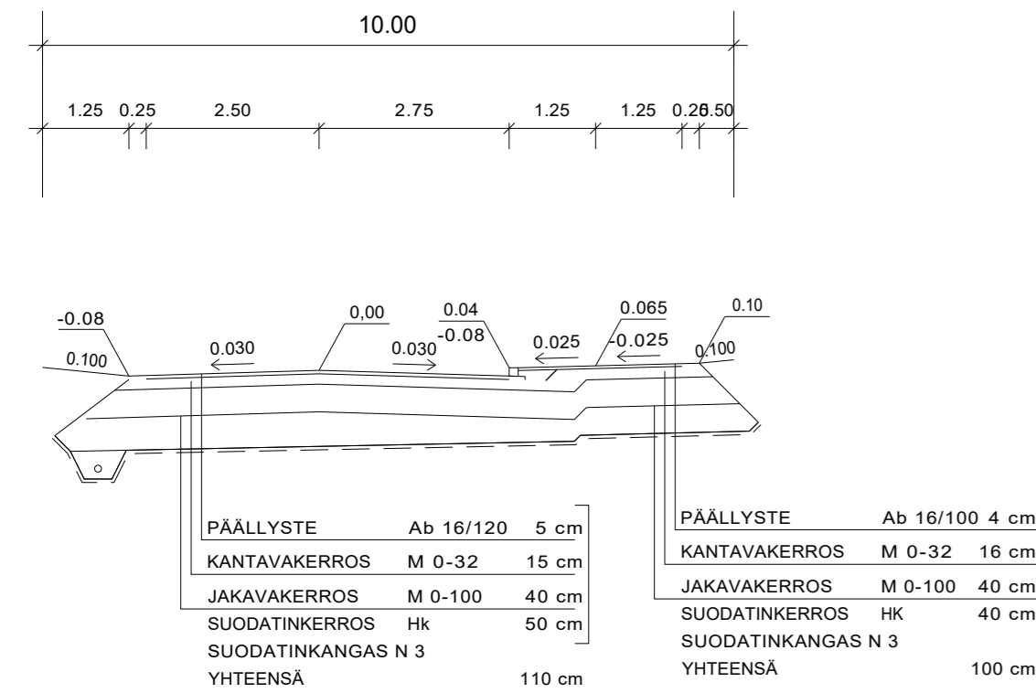
TYYPPIPOIKKILEIKKAUS PAALULTA 20 1:100
