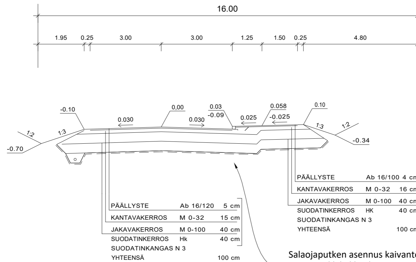
TYYPPIPOIKKILEIKKAUS PAALULTA 300 1:100
