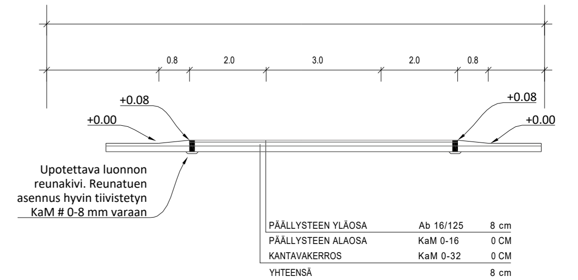
KOROTETTU SUOJATIE, TYYPPIPOIKKILEIKKAUS
