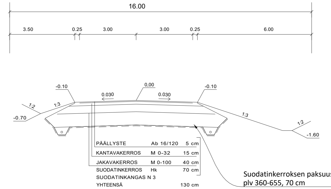
TYYPPIPOIKKILEIKKAUS PAALULTA 380 1:100
