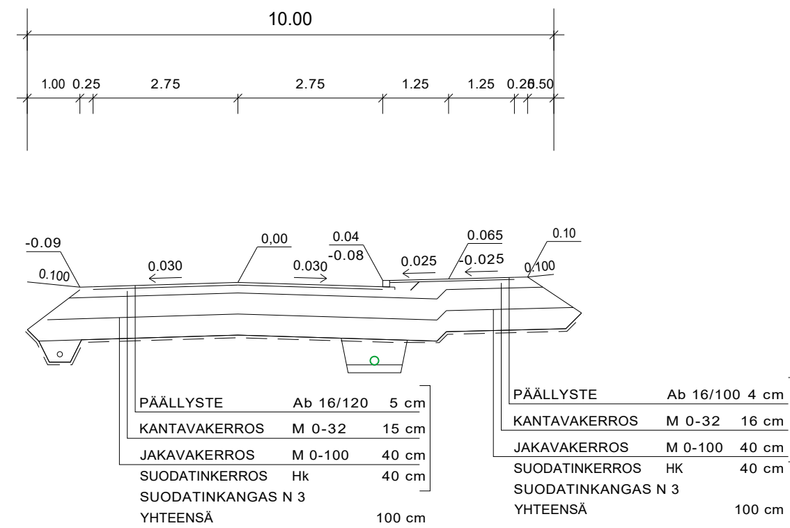
TYYPPIPOIKKILEIKKAUS PAALULTA 120 1:100
