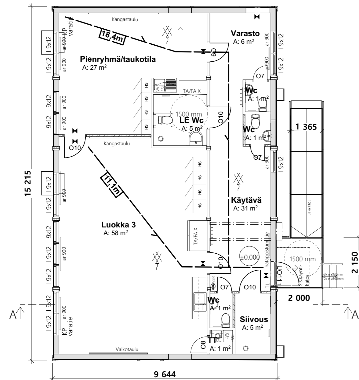
Pohjapiirros 1:100
